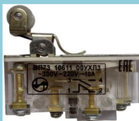
ВП73 10611 00УХЛЗ (с рычагом, аналог МП1107М)
