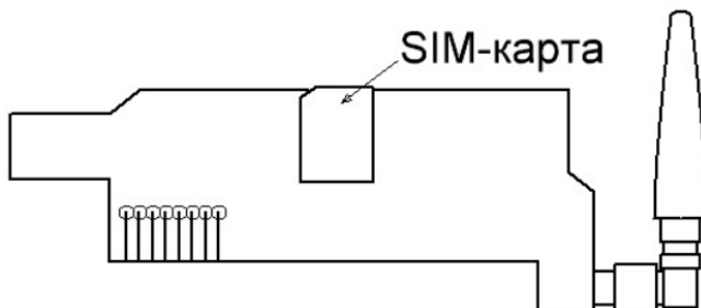
Рисунок 3 – Размещение SIM-карты в GSM-модуле
